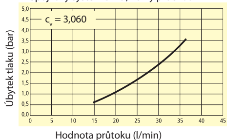
Graf průtoku vody* Spojkový systém DN 9, volný průchod
