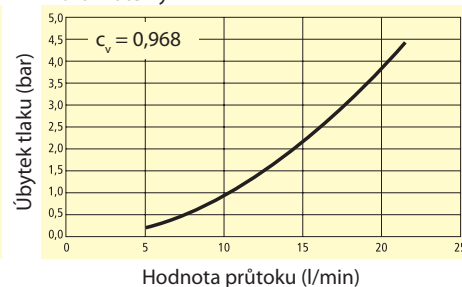
Graf průtoku vody* Spojkový systém DN 9, oboustranně uzavíratelný
