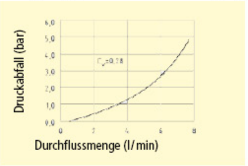
Durchflussdiagramm WASSER* Kupplungssystem ESME DN 5 beidseitig absperrend
