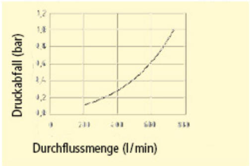
Durchflussdiagramm LUFT* Kupplungssystem ESME DN 5 einseitig absperrend
