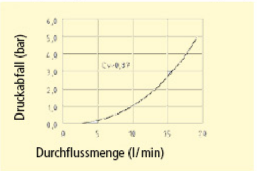
Durchflussdiagramm WASSER* Kupplungssystem ESME DN 5 einseitig absperrend
