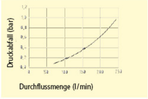
Durchflussdiagramm LUFT* Kupplungssystem ESME DN 5 beidseitig absperrend
