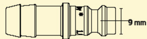
Steckprofil in Originalgröße
