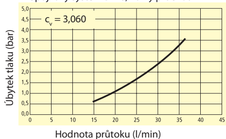
Graf průtoku vody* Spojkový systém DN 6, volný průchod
