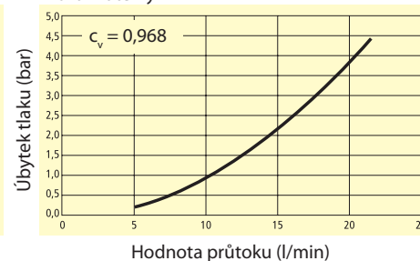
Graf průtoku vody* Spojkový systém DN 6, oboustranně uzavíratelný
