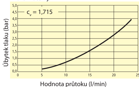
Graf průtoku vody* Spojkový systém DN 6, na jedné straně uzavíratelný
