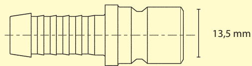
Profil vsuvky (originální velikost)
