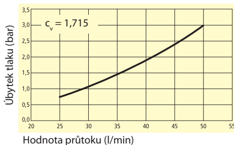
Graf průtoku vody* Spojkový systém DN 9, na jedné straně uzavíratelný
