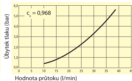
Graf průtoku vody* Spojkový systém DN 6, oboustranně uzavíratelný
